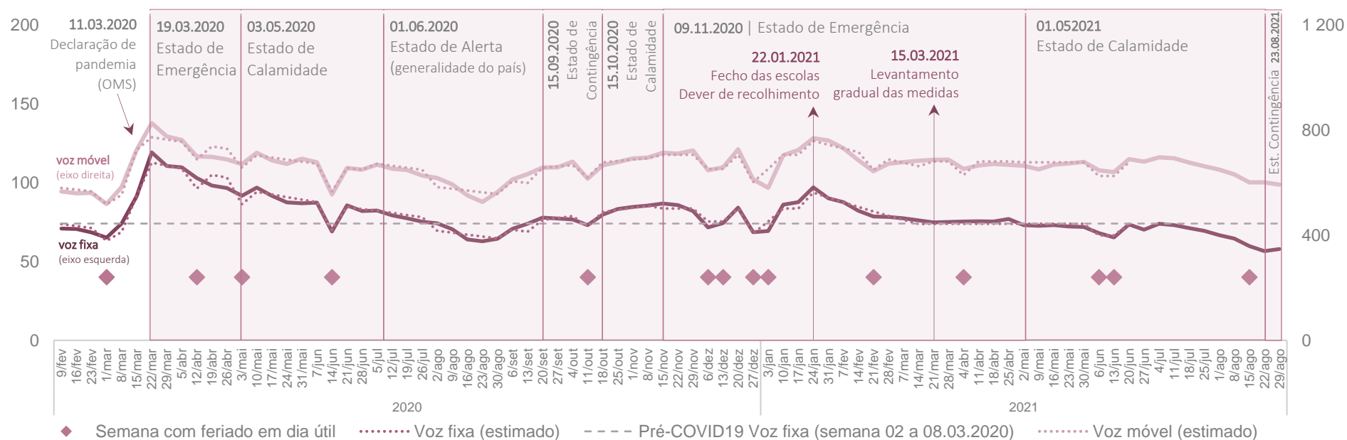
Figura 2 – Evolução semanal do tráfego de voz fixa e móvel desde fevereiro de 2020
